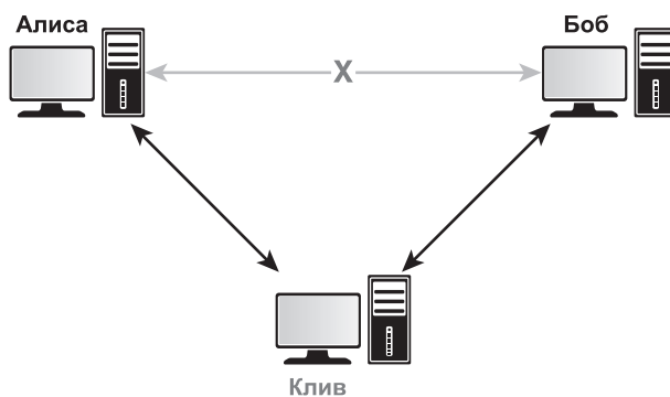
Рис. 10.1. Атака вида «незаконный посредник», в ходе которой Клив читает переписку между Алисой и Бобом
