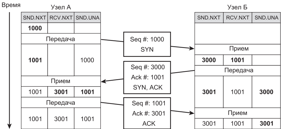
Рис. 2.13. Трехэтапное согласование
