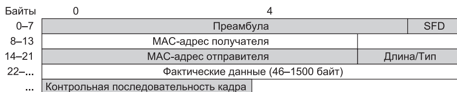
Рис. 2.4. Структура Ethernet-пакета
