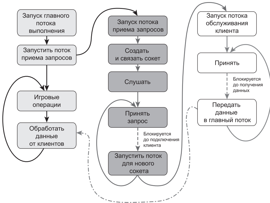
Рис. 3.1. Многопоточный процесс
